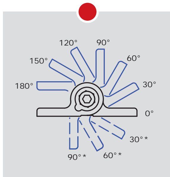
Einrastwinkelpositionen
